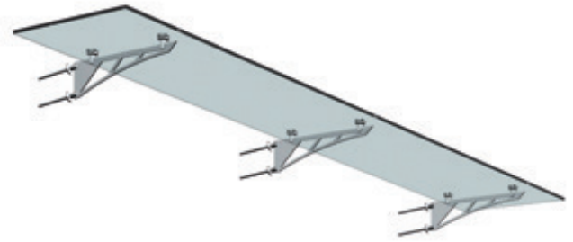
3 consoles pour longueur : 2400 mm
