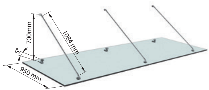
3 haubans pour longueurs : 2000-2400 mm
