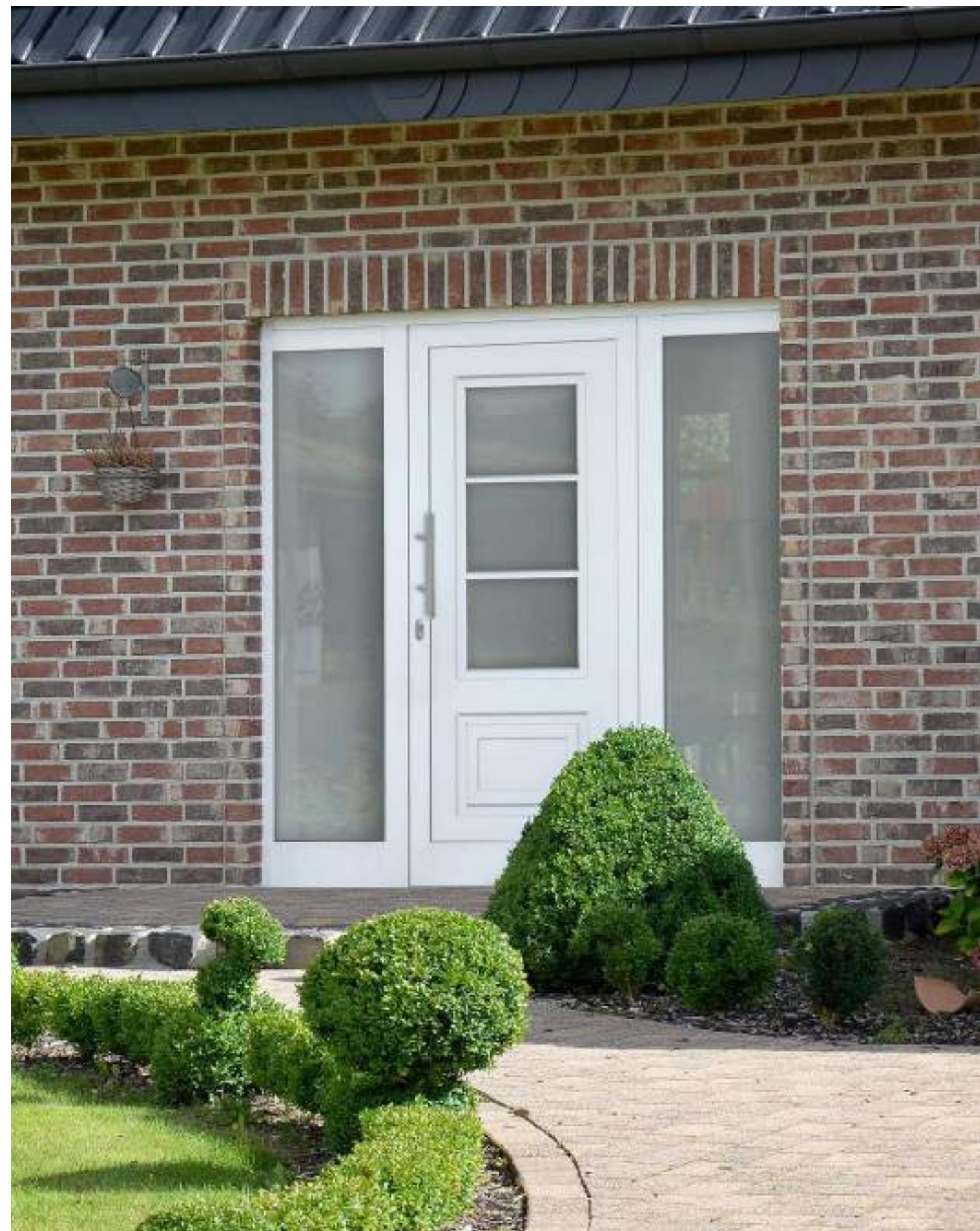
428-15 avec parties fixes | Couleur : blanc | Vitrage : Satinato | Poignée : 8.100.04.S inox | Type de pose : en feuillure ID porte : P24-428-15h
